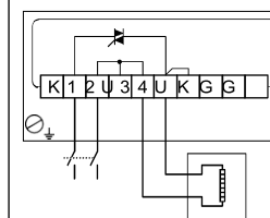
Figur 1 Inkoppling av matningsspänning och belastning, med skruvplint att koppla till jord och vidare till inkopplad värmelast.
