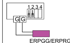
Figur 3 Omkopplarinställning och anslutning för internt börvärde och extern givare.
